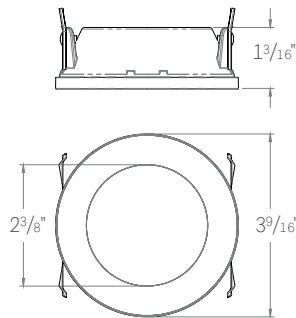
ED3-RFTL ROUND FIXED TRIMLESS
